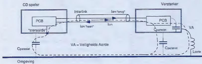
Figuur 3 CM en DM stromen
